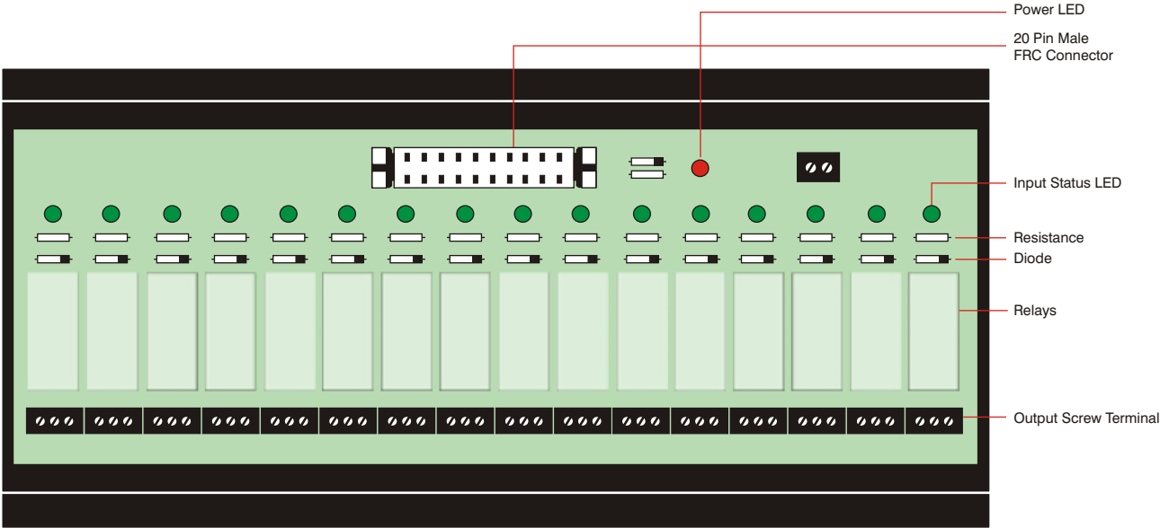
Layout of TT-IMRB-16024D1S-DO(F20)
