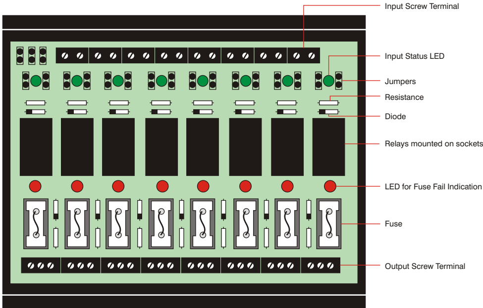
Layout of TT-IMRB-08024D1S-CSSRFFI(EL-5A)
