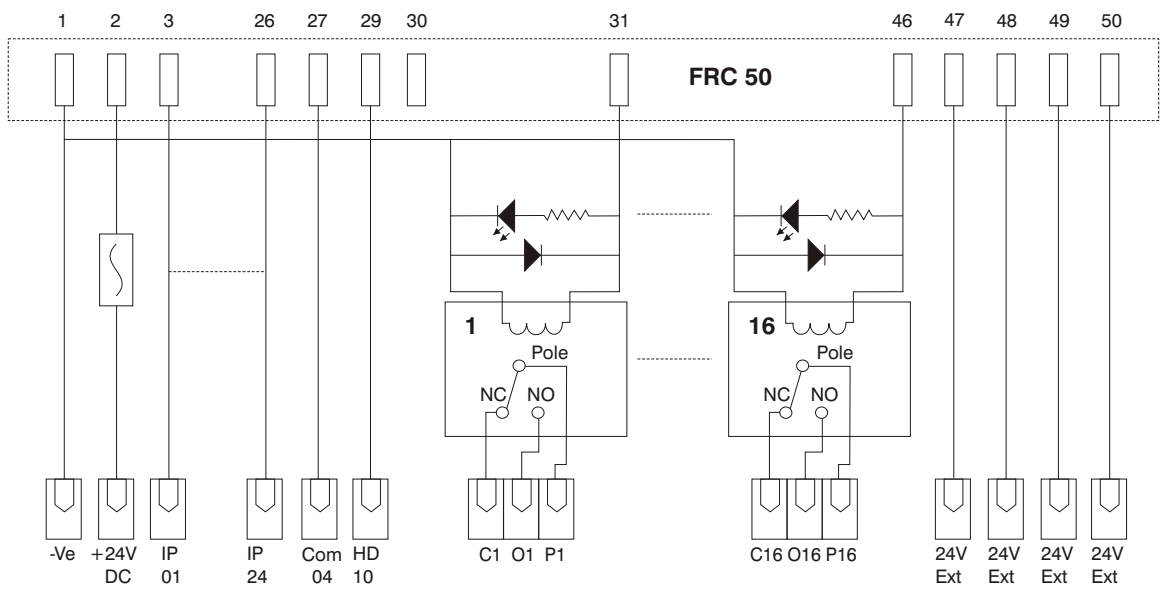
Schematic of TT-IMRB-16024D1S-CNC
